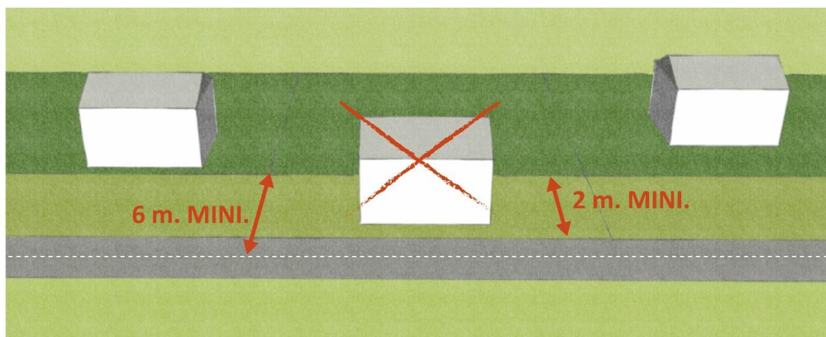
Schéma d'implantation
